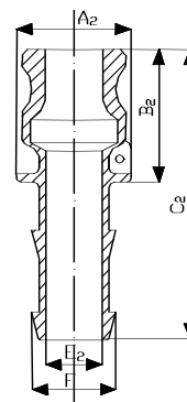
TÖMLŐCSONKOS APA E TÍPUS
