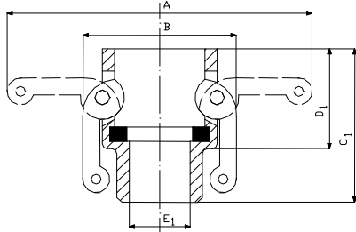
HEGTOLDATOS ANYA BW TÍPUS
