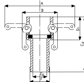
TÖMLŐCSONKOS ANYA C TÍPUS
