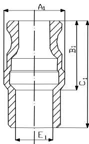
HEGTOLDATOS APA FW TÍPUS
