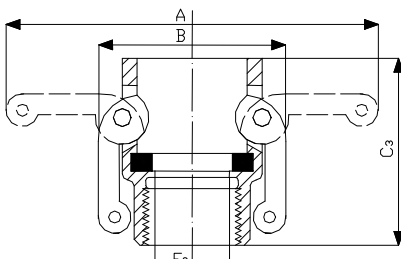
MENETES ANYA D TÍPUS
