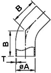
BPE 45° Elbow Weld End (DT-8)
